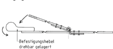
Befestigungshebel "Vorreiber"
